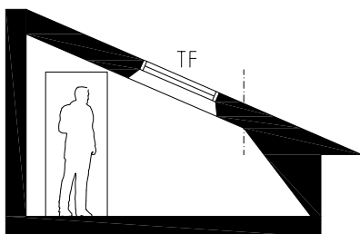
SEKTION GENOM PLAN 3 TR
